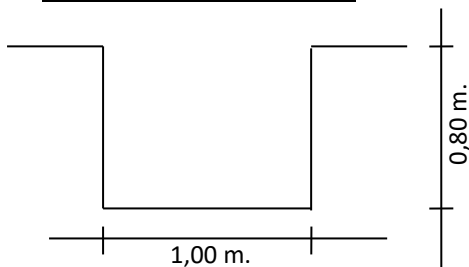
CANAL LA CAÑADA
