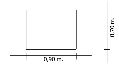
CANAL CUATRO CHICO
