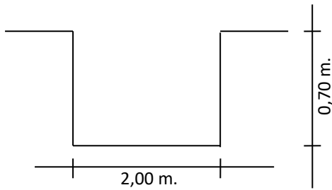
CANAL GRAL. CERRO NEGRO
