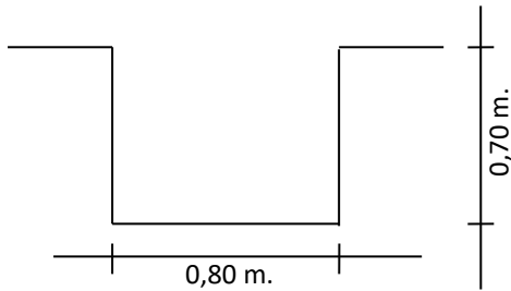
CANAL CUATRO GRANDE
