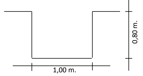
CANAL LAS LOMITAS
