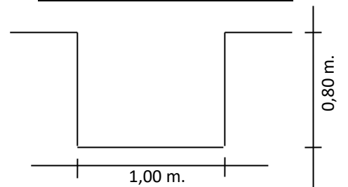
CANAL CERRO NEGRO
