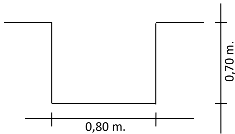
CANAL BAJO ANGUALASTO
