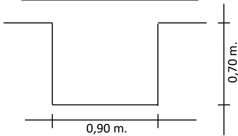
CANAL COLONIA DOS
