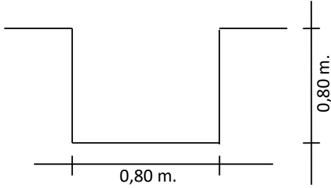
CANAL ARROYITO LAS FLORES
